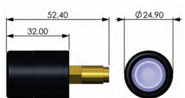
Light (AC-LED-001A)
